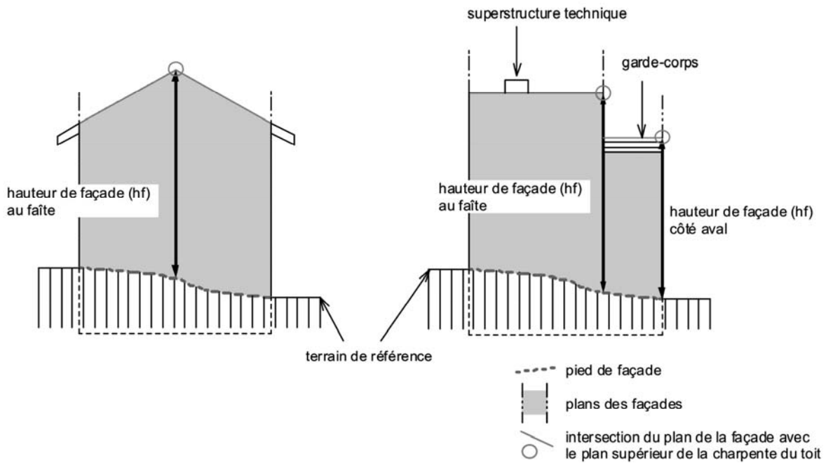
Figure 4.2.b Hauteur de façade
