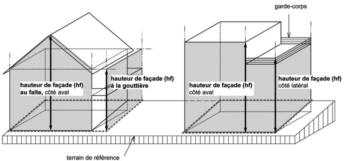
Figure 4.2.a Hauteur de façade
