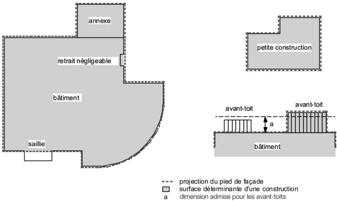
Figure 7.4 Surface déterminante d'une construction
