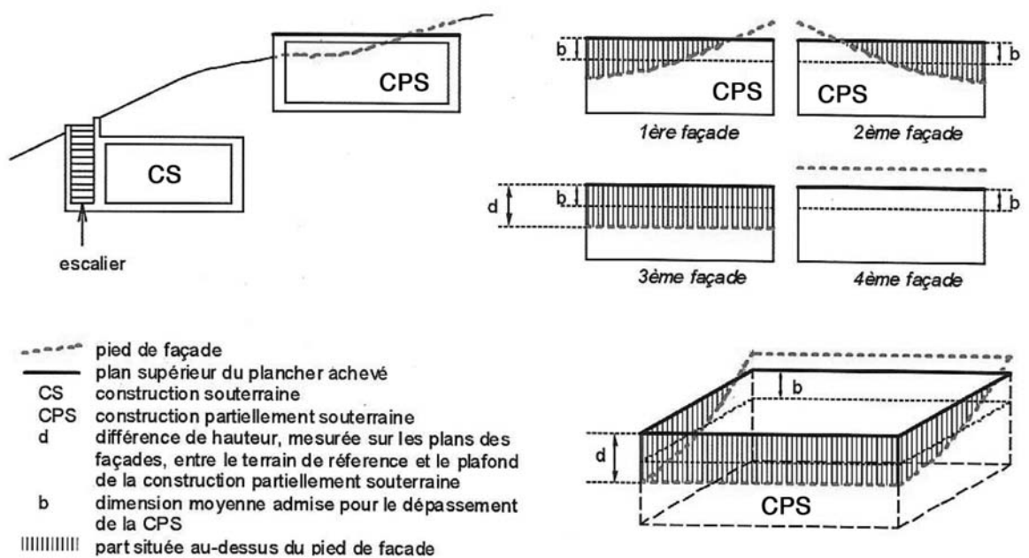
Figures 1.3 et 1.4 Constructions souterraines, constructions en sous-sol
