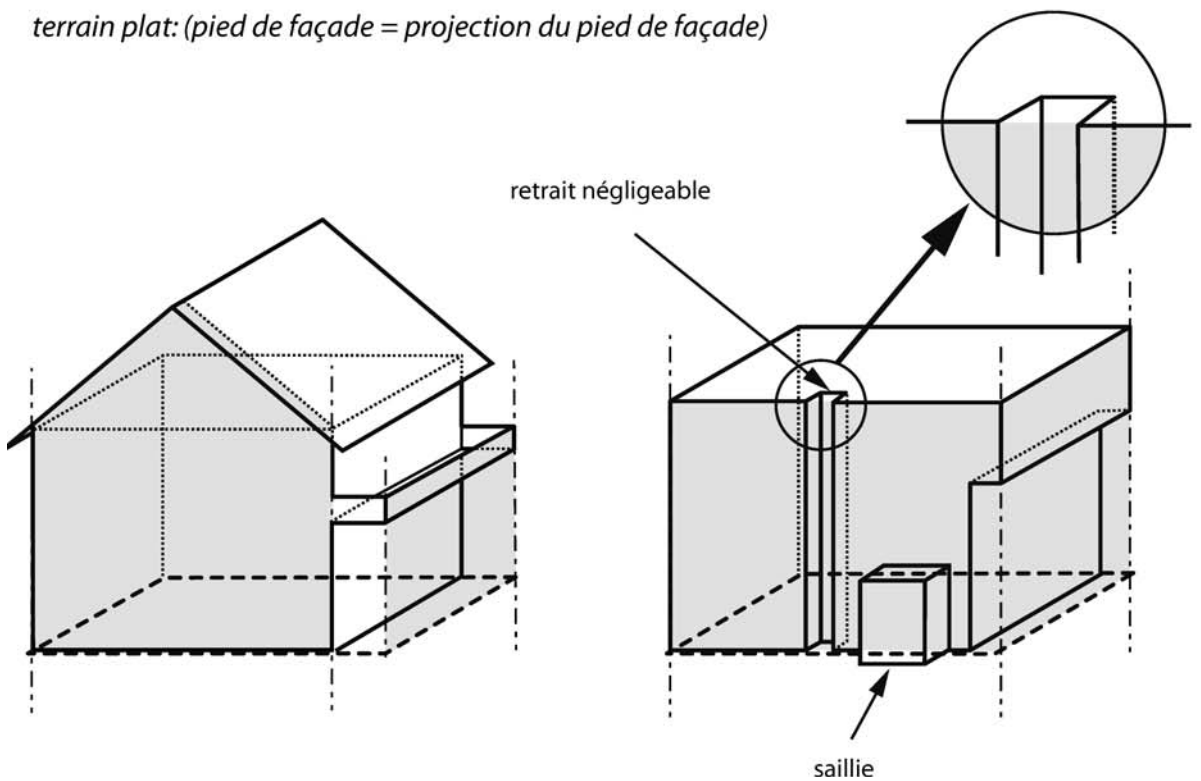
Figure 2.2a Plan de façade et projection du pied de façade (sur terrain plat)
