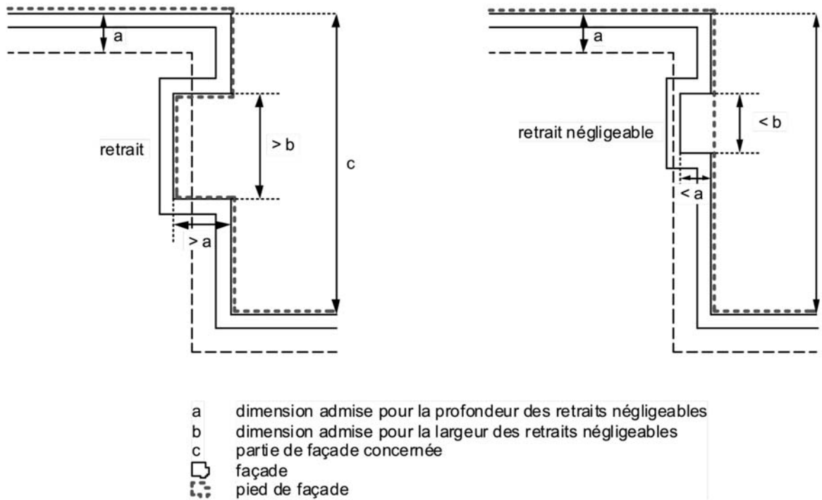
Figure 2.4 Retraits et retraits négligeables
