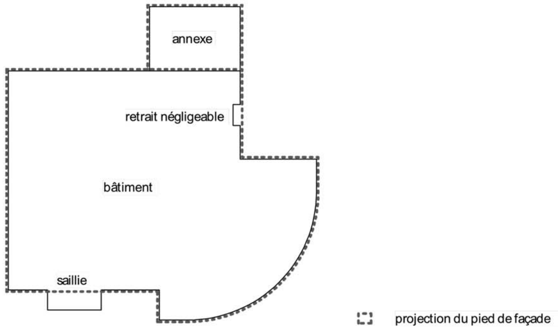
Figure 2.1 Projection du pied de façade
