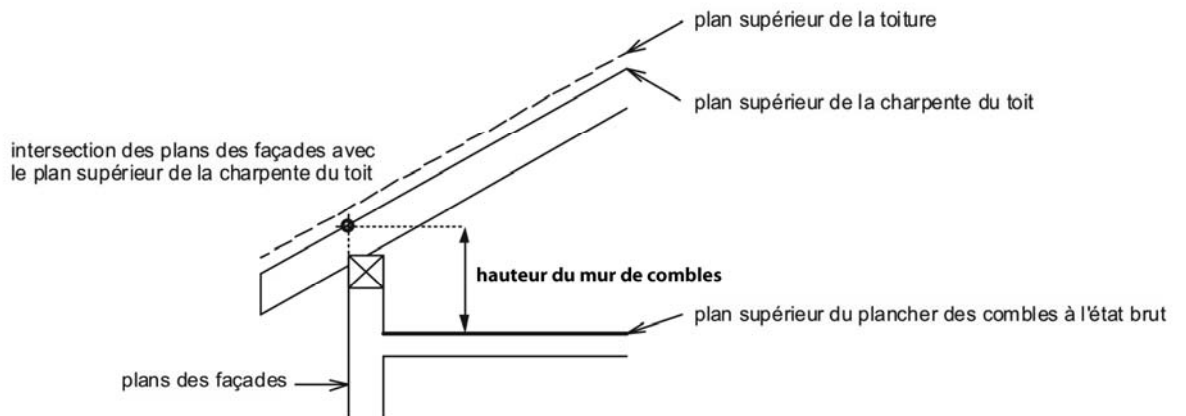
Figure 4.3 Hauteur du mur de combles
