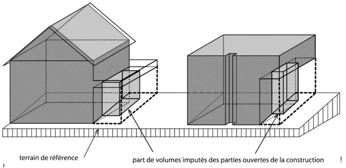
Figure 7.3 Indice de masse
