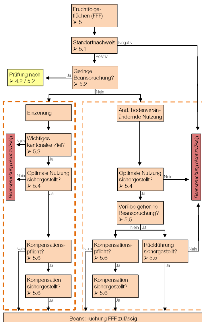
Abbildung 5 Entscheidungsbaum FFF
